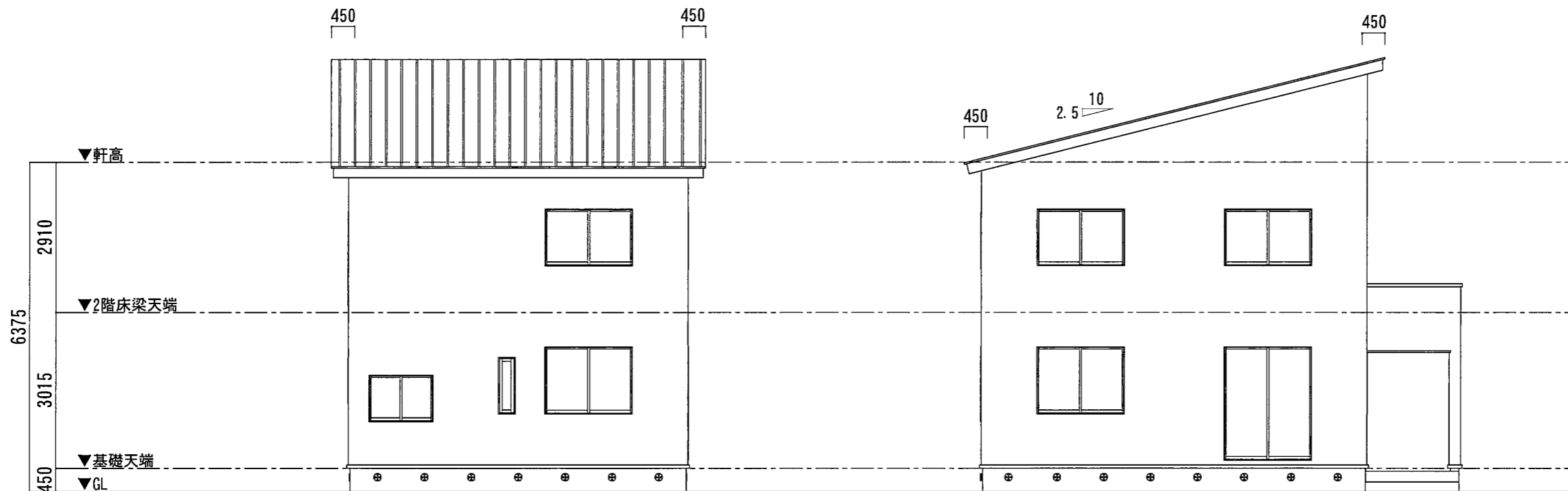
側立面図
