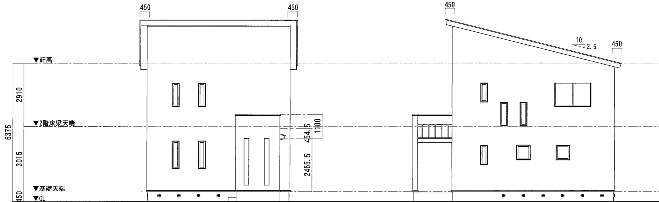
側立面図
