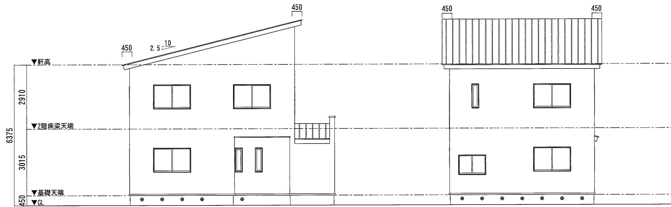
側立面図
