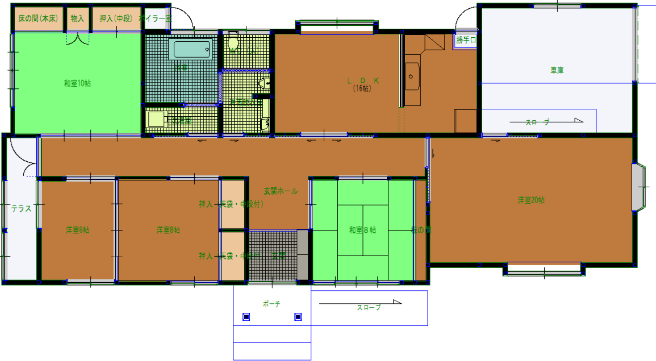
1 階平面図
