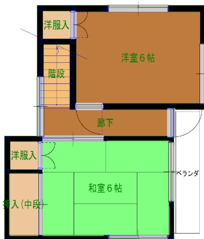
2階平面図
