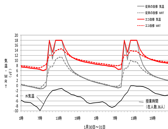
冬季の気温、MRT、暖房負荷の経時変化 (プランB Ⅱ地域)
