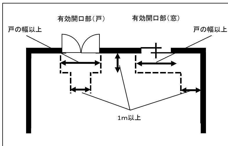
《室内に確保する通路の例》
