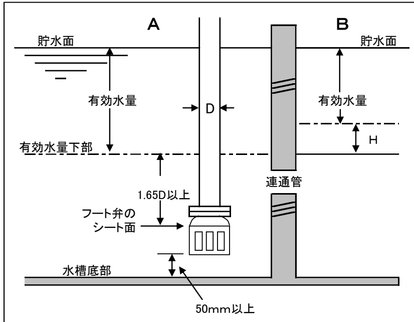
《サクシオンピットを設けない場合又は連通管を設ける場合の例》
